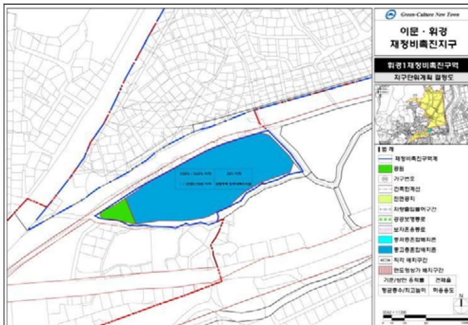
[지구단위계획 결정도(변경없음)]
