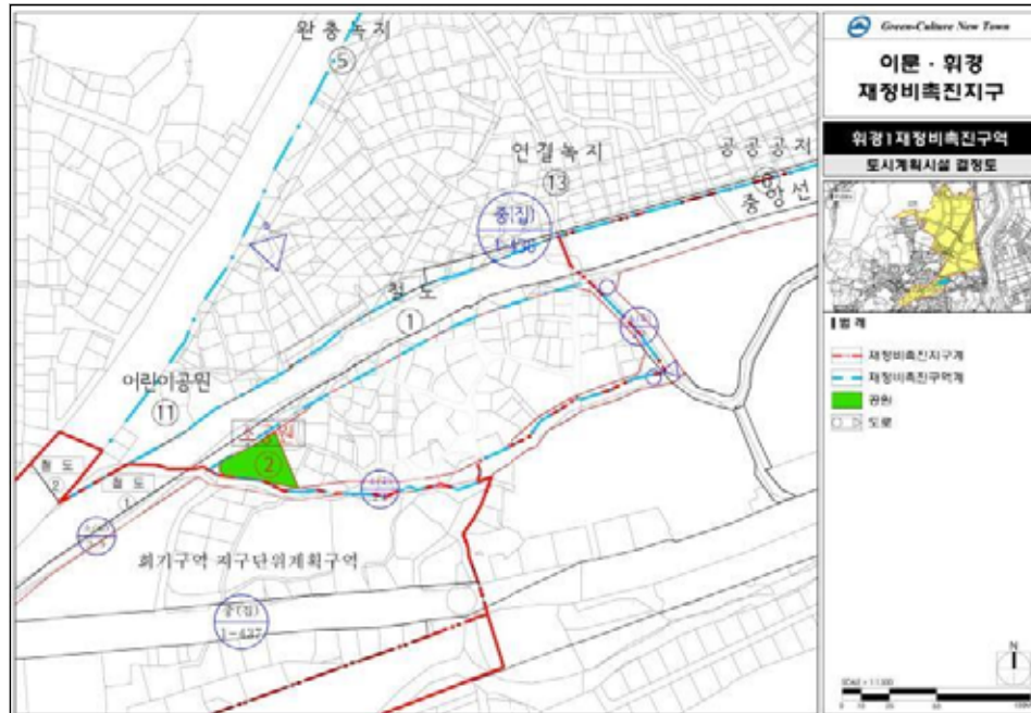
[도시계획시설 결정도(변경없음)]
